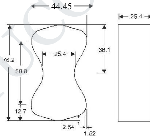
Fig. 31 Dimensions of Standard Briquette
