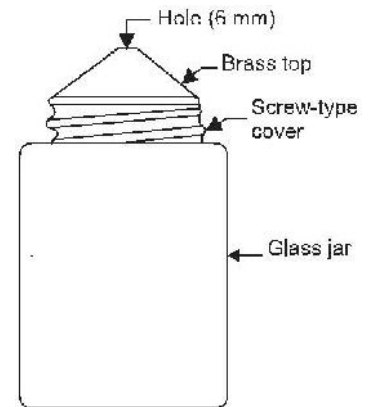
Fig.37 Pycnometer
