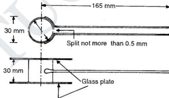
Fig. 30 Le-chatelier Apparatus
