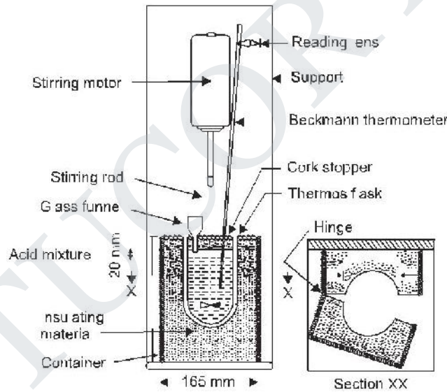
Fig. Calorimeter
